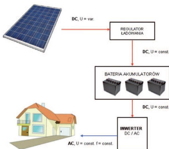
Rysunek 23 Schemat instalacji mieszanej 193 (oznaczenia: DC- prąd stały, AC-prąd przemienny, U- napięcie, f-częstotliwość, var.-zmienne, const.- stałe)
