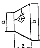
Rys. 1 Kształt płyt sześciokątnych
