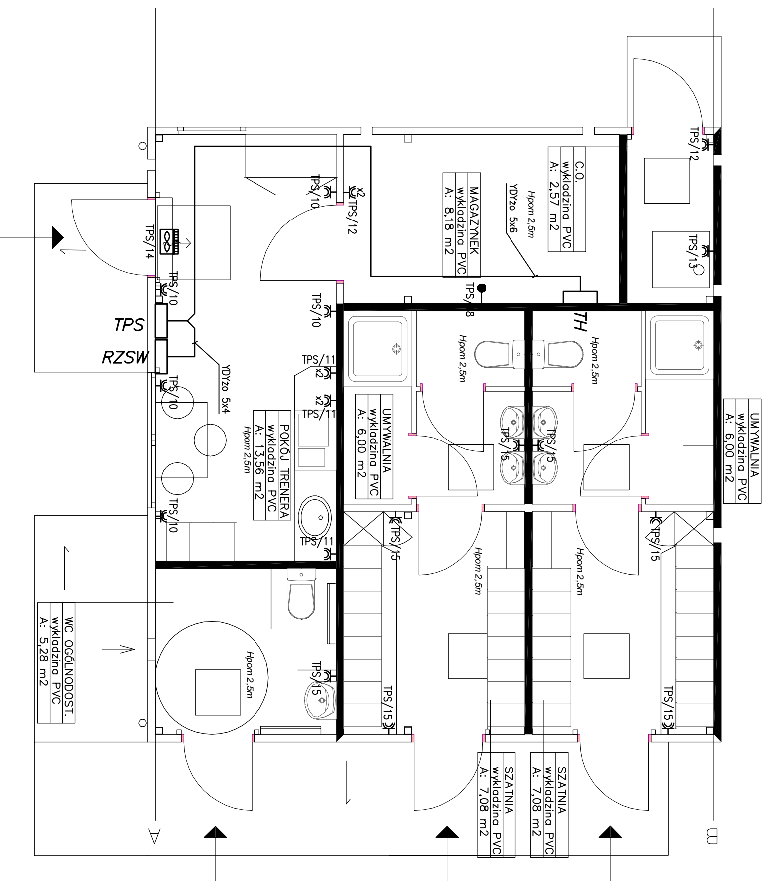
RZUT PRZYZIEMI
