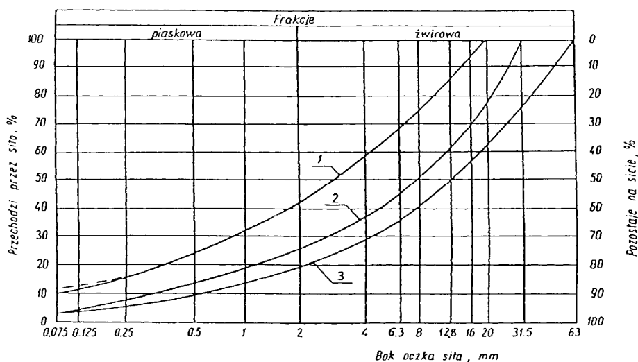
Rysunek 1. Pole dobrego uziarnienia kruszyw przeznaczonych na podbudowy wykonywane metodą stabilizacji mechanicznej: 1-2 kruszywo na podbudowę pomocniczą (dolną warstwę).
