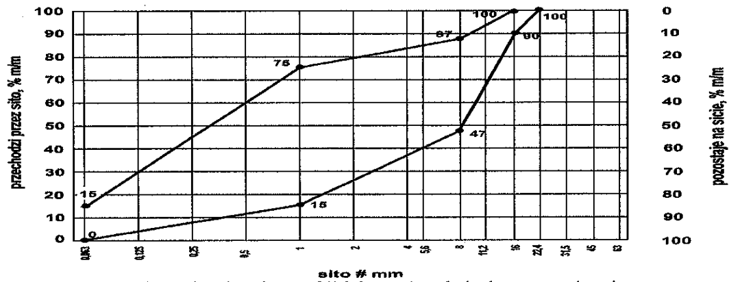
Rys. 17. Mieszanka niezwiązana 0/16 do nawierzchni z kruszywa niezwiązanego
