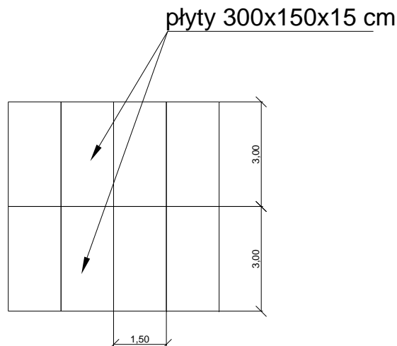
Rys.2. Schemat układania płyt
