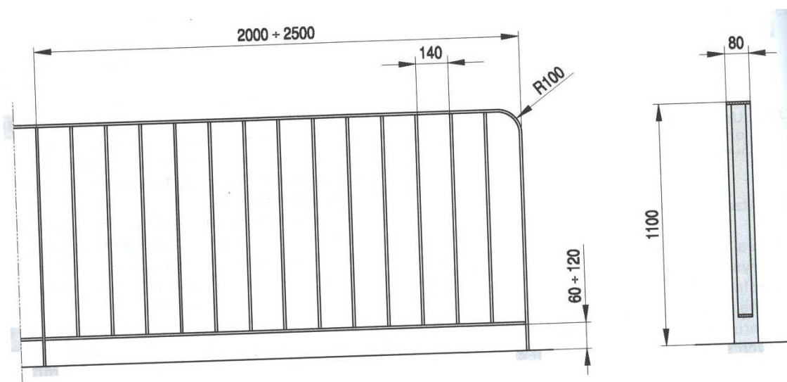
Rys. nr 1 Przykład balustrady U-11a
