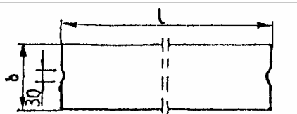
Rys. 1. Wymiarowanie krawężników
