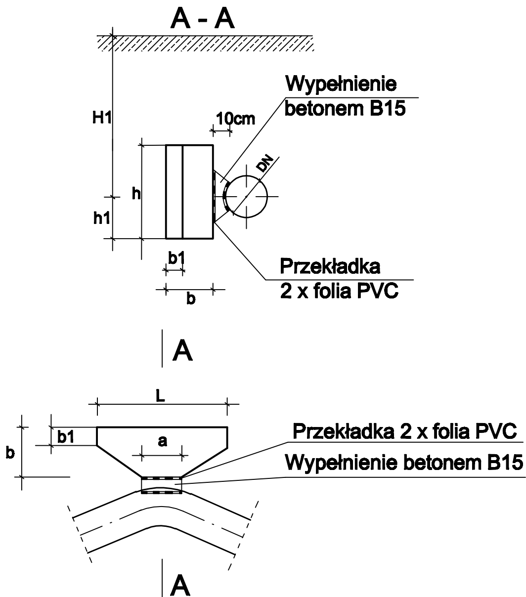
WYMIARY BLOKÓW OPOROWYCH [m]
