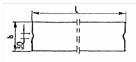
Rys. 1. Wymiary krawężników
