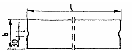
Rys. 1. Wymiarowanie krawężników
